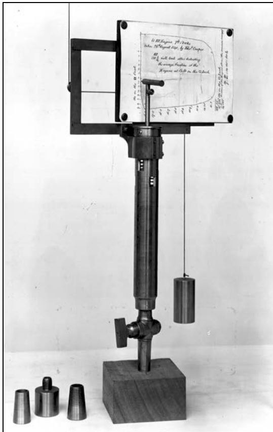
Abb. 2.35: „Watt-Indikator“ zur automatischen Aufzeichnung der Volumen-Druck-Kurve bei einer Dampfmaschine
