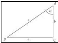
Abb. 2.8: Dreieck als Grund- lage v. Plimpton 322
