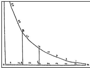
Abb. 2.25: Lebenserwartungskurve von HUYGENS
