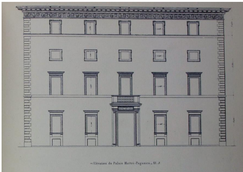
Abb. 17: Palazzo Mattei di Paganica, Fassade nach Létarouilly
