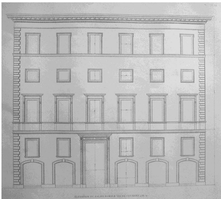
Abb. 34-35: Palazzo Ruggieri, Fassade nach Létarouilly und Detail
