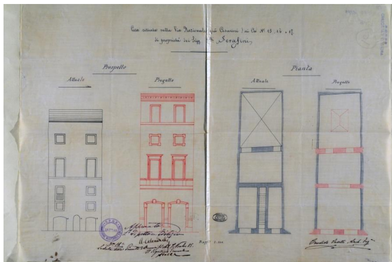
Abb. 36-37: Palazzo Ruggieri, Projekt zur Angleichung des benachbarten Gebäudes, 1886, und Detail
