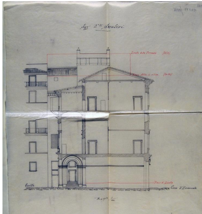
Abb. 39: Palazzo Ruggieri, Projekt für ein Attikageschoss, 1886
