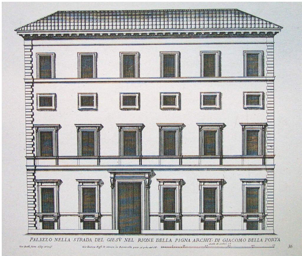
Abb. 11: Palazzo Ruggieri, Fassade nach Falda
