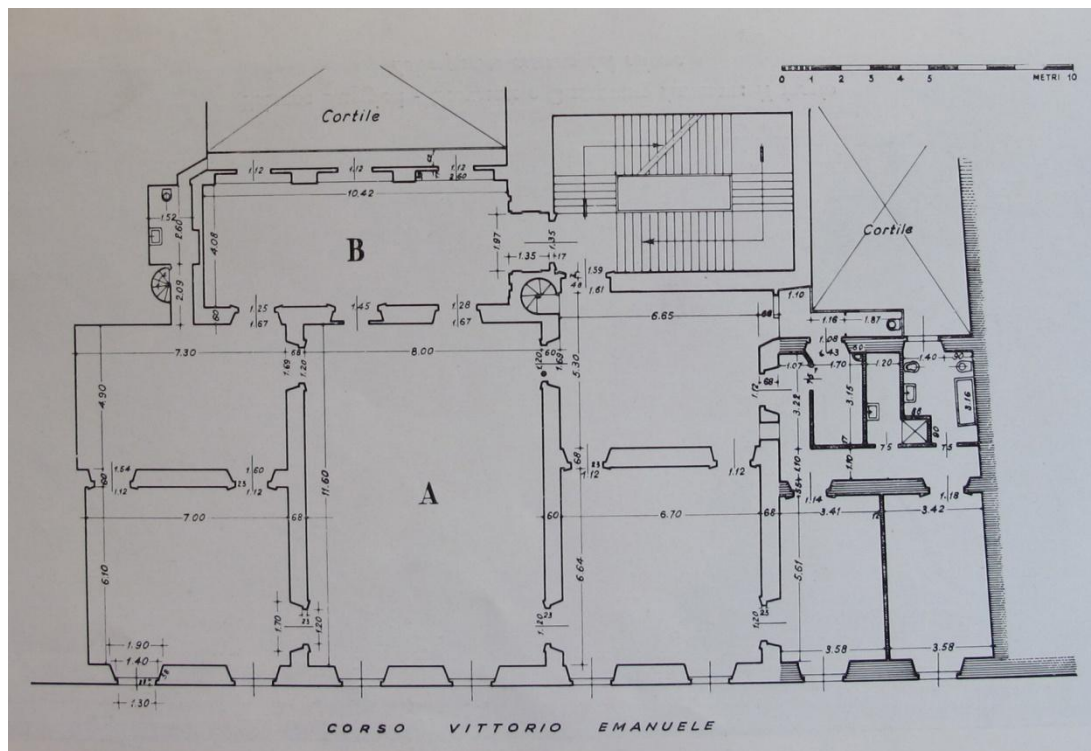
Abb. 6: Palazzo Ruggieri, Piano Nobile, Grundriss
