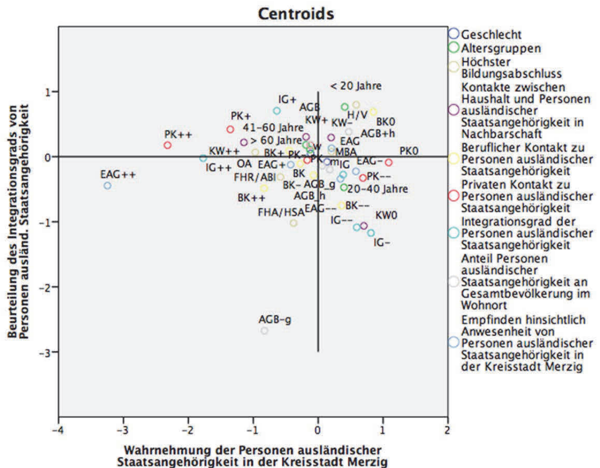
Abbildung 80: Kanonische Korrespondenzanalyse 3
